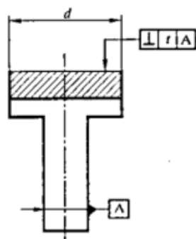
图 4 一垂直度公差的标注示例
