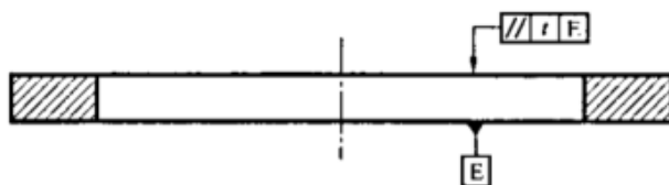
图 3 —平行度公差标注示例:挤出型材的切割产品
