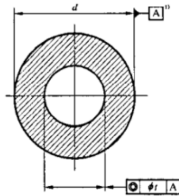
图 6 芯轴支撑的压出制品的同轴度公差标注示例
