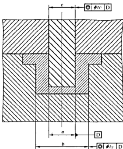
图 5 模压制品同轴度公差标注示例
