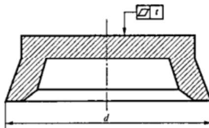
图 1 一平面度公差标注示例
