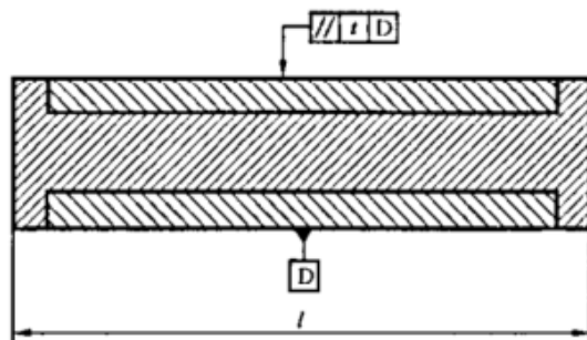
图 2 —平行度公差标注示例:夹层结构
